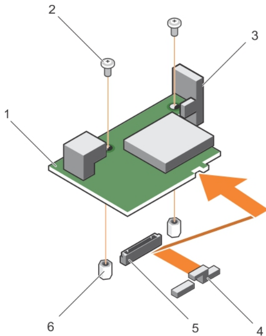
Abbildung 24. Entfernen der IDSDM-Karte
