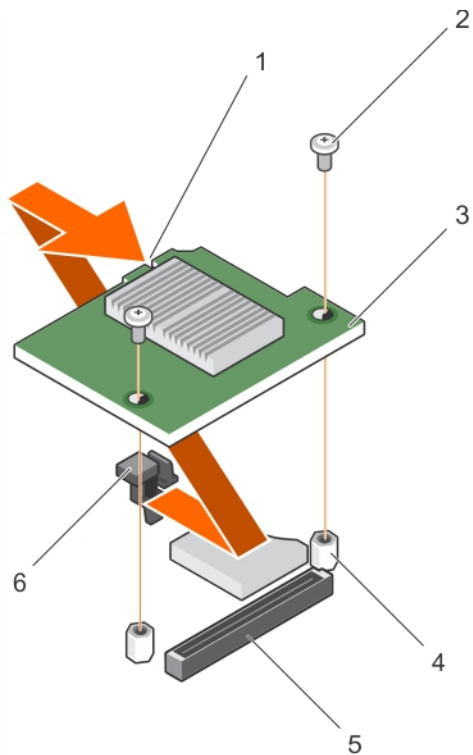
Abbildung 30. Entfernen der NDC
