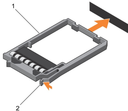
Abbildung 47. Installieren eines 1,8-Zoll-SSD-Platzhalters
