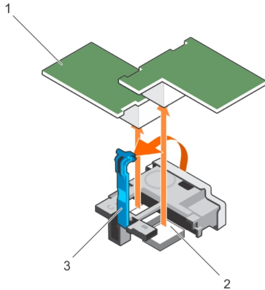
Abbildung 17. Entfernen einer PCIe-Mezzaninekarte
