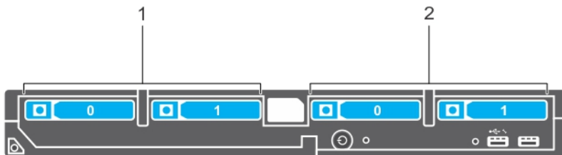
Abbildung 38. Festplatten- oder SSD- und PCIe- SSD-Schachtnummerierung – 2,5-Zoll-Festplatten- oder -SSD- und PCIe-SSD-System
