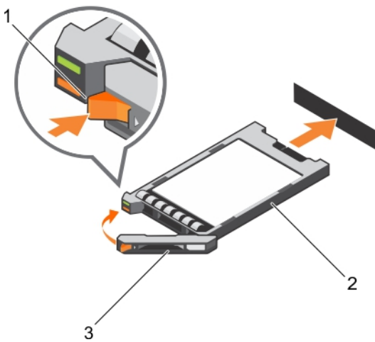
Abbildung 43. Installieren eines SSD
