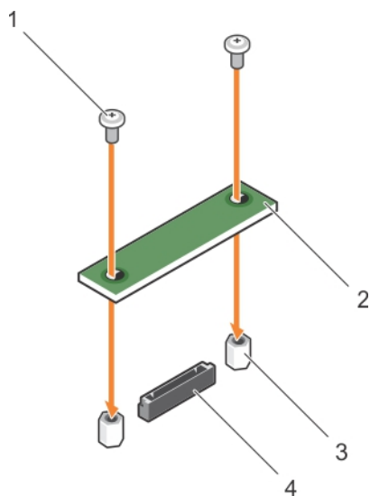
Abbildung 27. Installieren der rSPI-Karte
