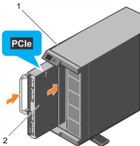
Abbildung 7. Installieren eines Servermoduls
