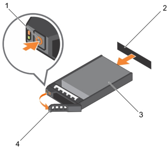
Abbildung 40. Entfernen eines Laufwerks
