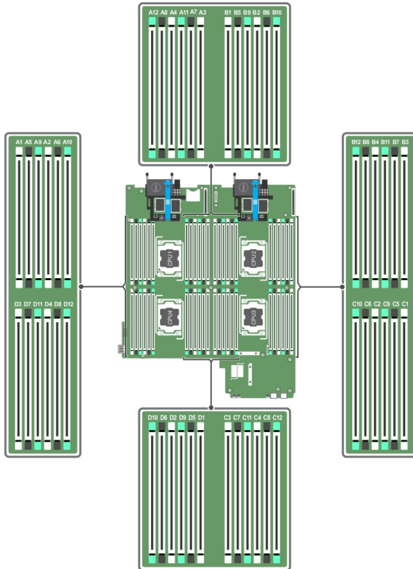
Abbildung 14. Positionen der Speichersockel
