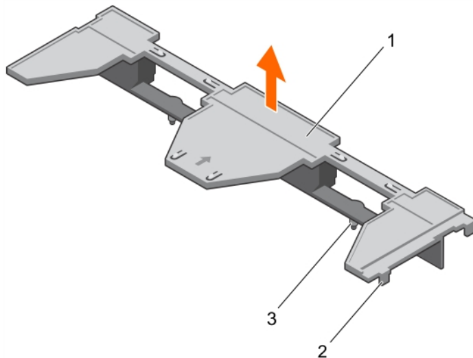
Abbildung 11. Entfernen des Kühlgehäuses
