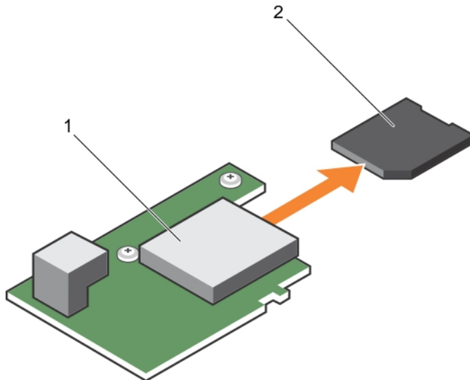
Abbildung 21. Austauschen einer SD-Karte
