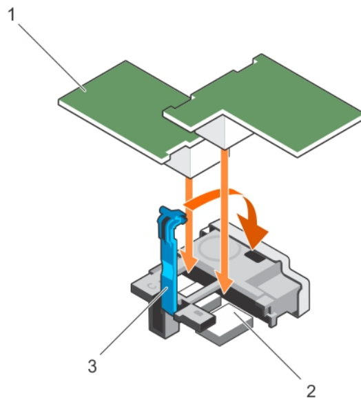
Abbildung 18. Installieren einer PCIe-Mezzaninekarte
