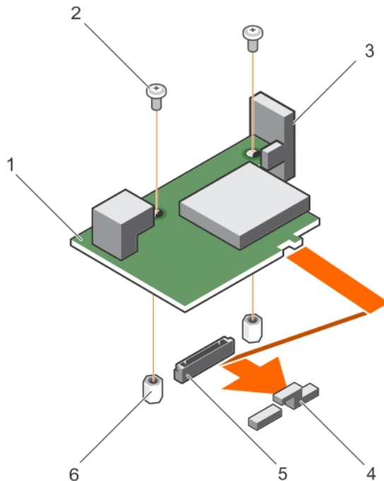
Abbildung 25. Installieren der IDSDM-Karte
