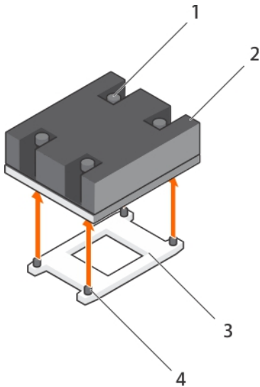
Abbildung 32. Entfernen des -Kühlkörpers
