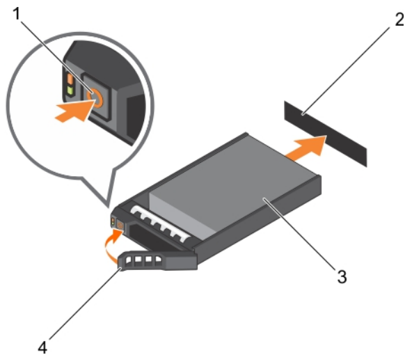
Abbildung 42. Einbauen eines Laufwerks
