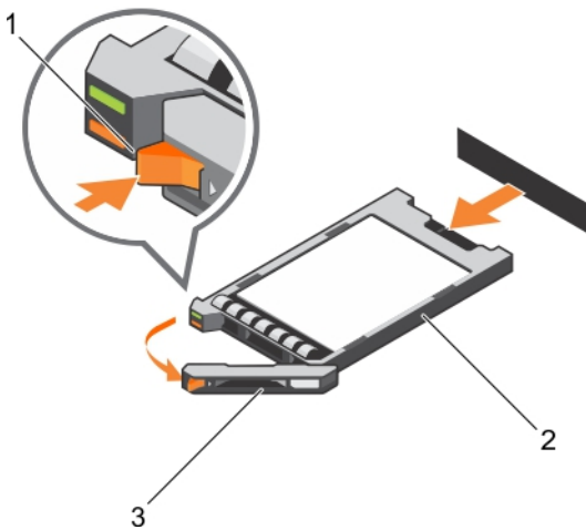
Abbildung 41. Entfernen eines SSD-Laufwerks
