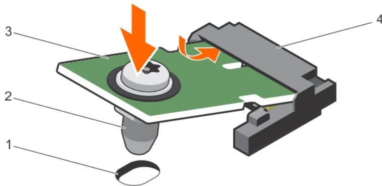
Abbildung 71. Einsetzen des TPM
