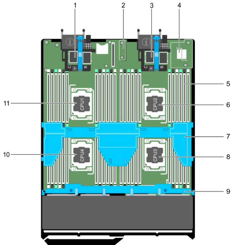
Abbildung 10. Im Inneren des Servermoduls
