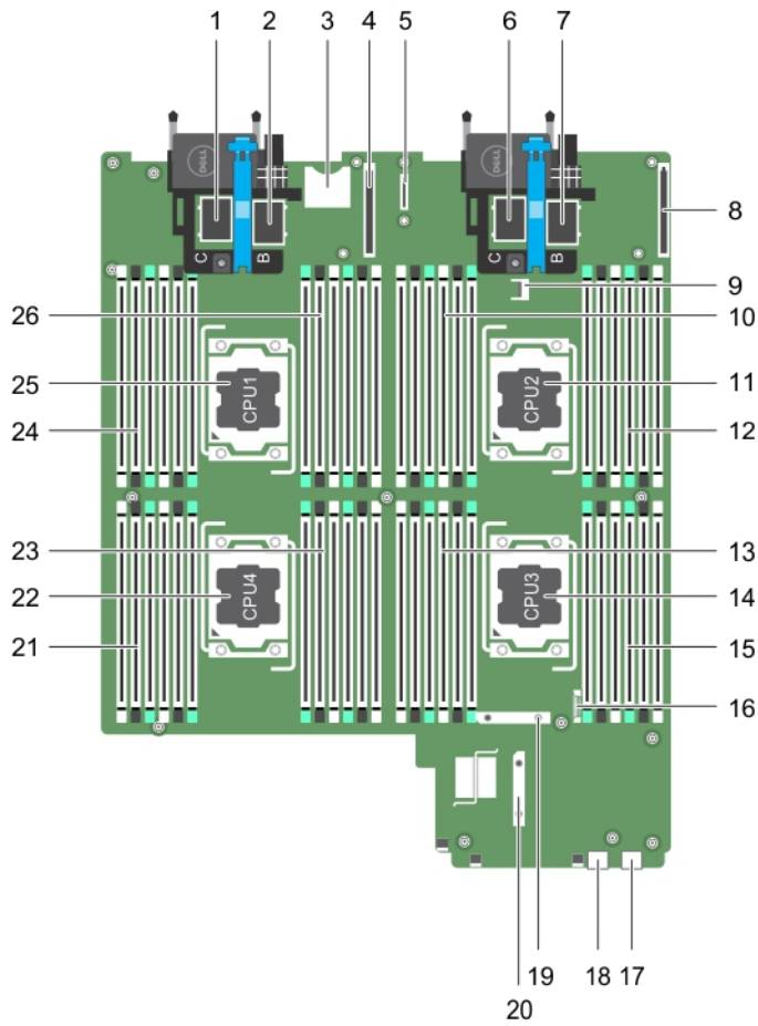
Abbildung 72. Systemplatinenanschlüsse
