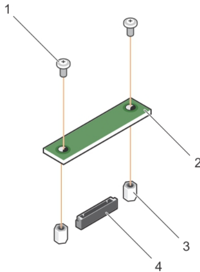
Abbildung 26. Entfernen der rSPI-Karte
