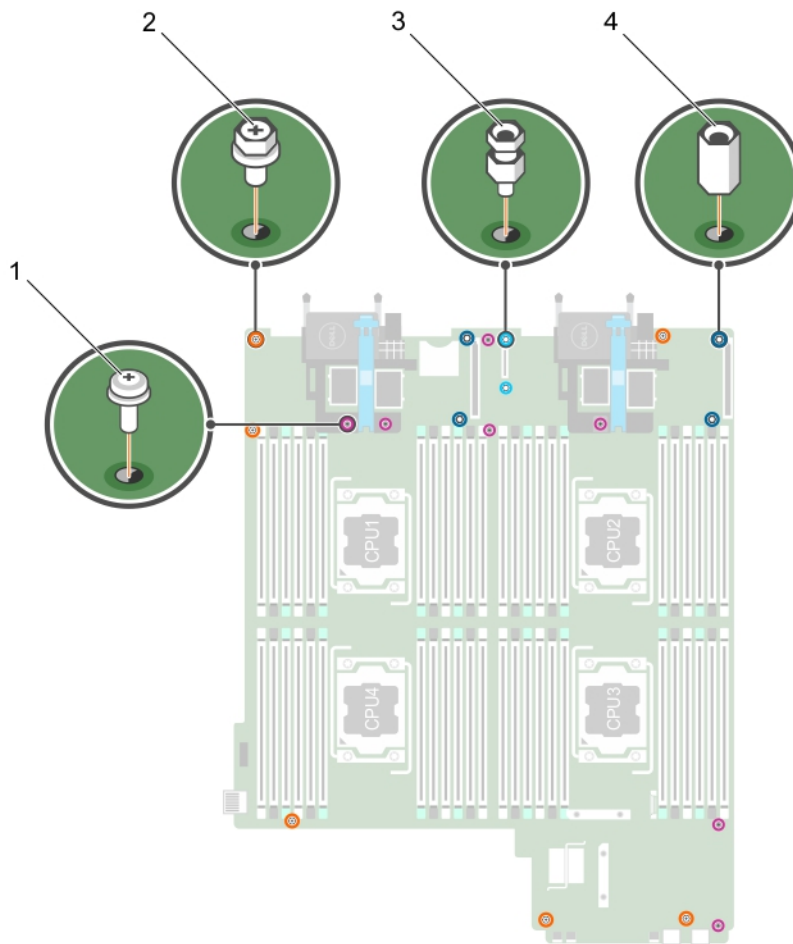
Abbildung 68. Verschiedene Arten von Schrauben auf der Systemplatine
