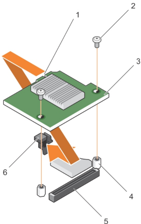
Abbildung 31. Installieren der NDC
